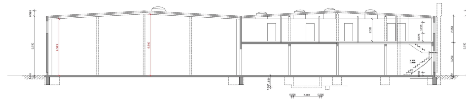
SCHNITT A-A
